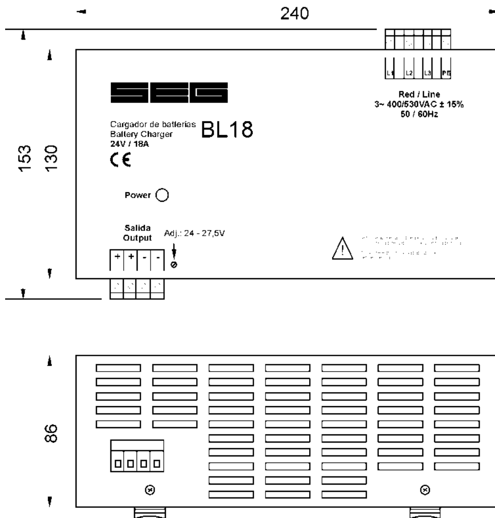
Figura 4.1: Dimensiones de la caja
