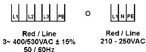
Figura 3.2: Conexión a la red
