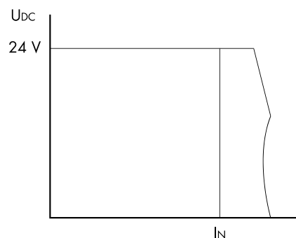
Figura 3.3: Limitación de corriente
